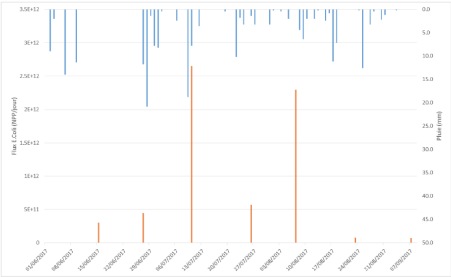
Figure 16 : Flux en E. coli du ru de Chantereine pendant l'été 2017 et cumul journalier de précipitations (pluviomètre GY28, DEA93).
