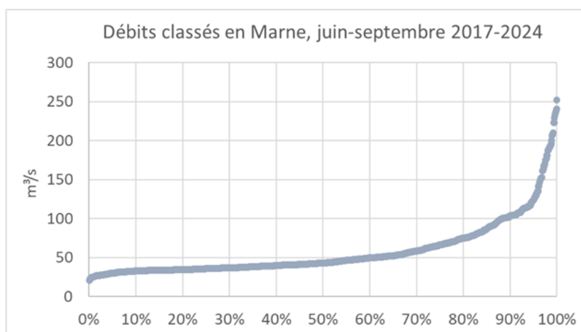
Figure 7 : Débits classés de la Marne sur la période estivale des années 2017 à 2024.
