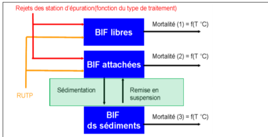
Figure 27 : Schéma des processus modélisés par WAQTEL.
