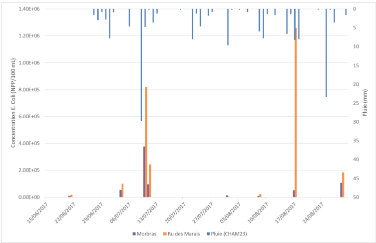
Figure 17 : Concentrations en E. coli (ru des Marais et Morbras) et cumul journalier des précipitations (pluviomètre CHAM23, DSEA).
