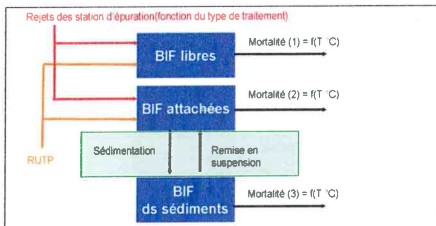
Figure 28 : Schéma des processus modélisés par WAQTEL.
