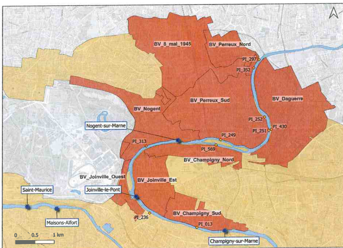
Figure 30 : Secteur caractérisé par un manque d'apports bactériologiques de temps sec et localisation des apports supplémentaires estimés.
