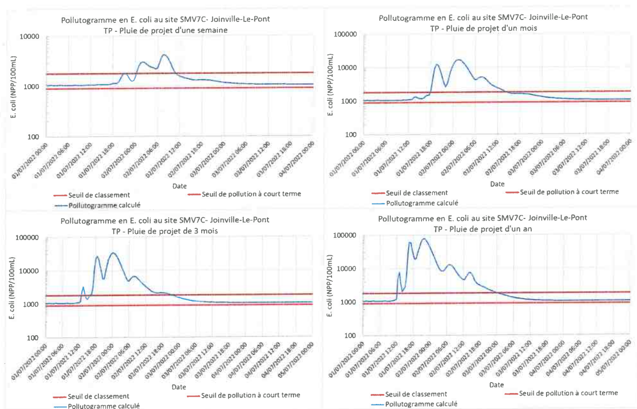
Figure 37 : Pollutogrammes simulés pour les pluies de projet au site de Joinville-le-Pont ( E. coli ).
