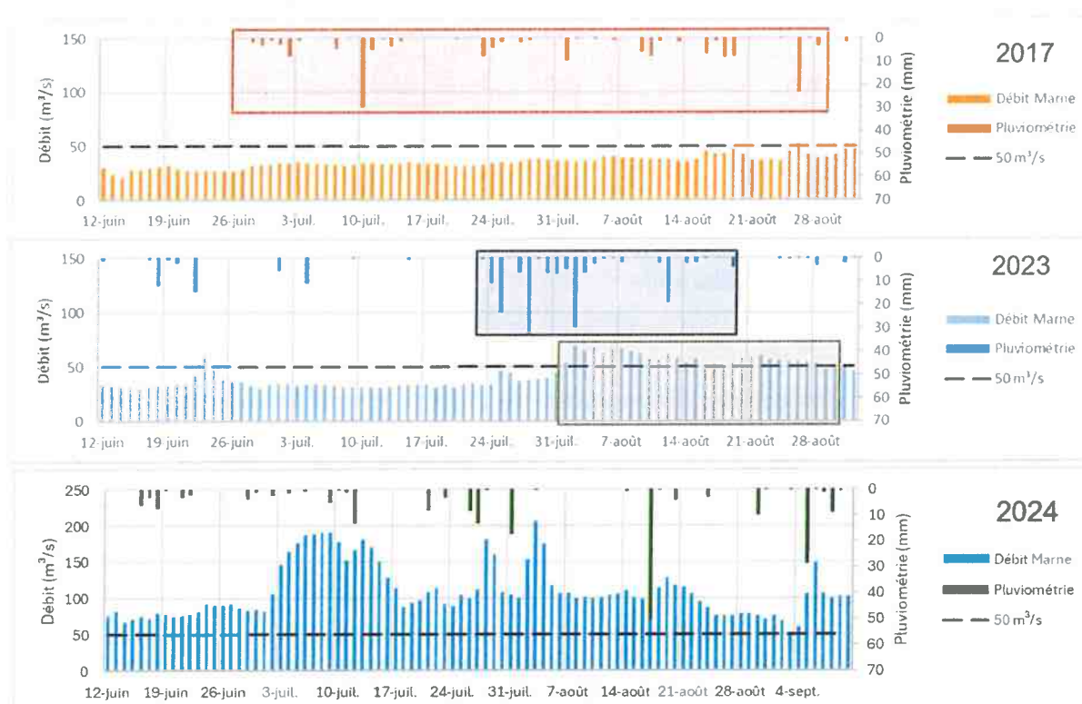
Figure 12 : Comparaison de la pluviométrie et des débits en 2017, 2023 et 2024.
