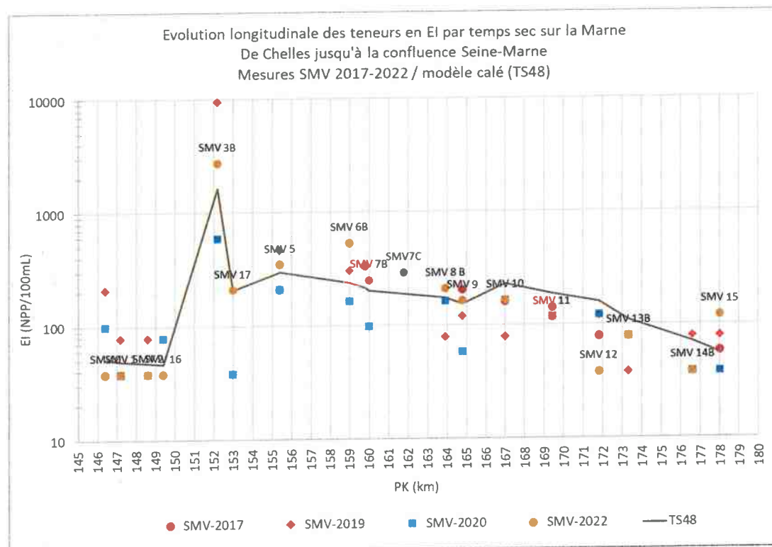
Figure 32 : Comparaison des résultats du modèle EI calé en temps sec aux données SMV
