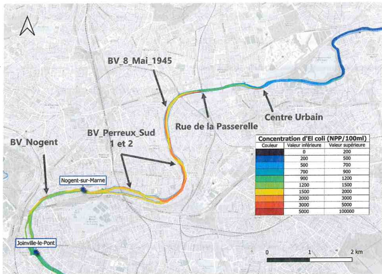
Figure 35: Simulation de la qualité bactériologique de la Marne par temps sec en amont du site de Joinville-le-Pont
