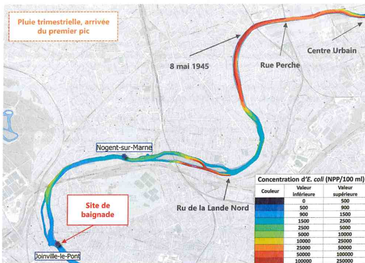
Figure 36: Simulation de la qualité bactériologique de la Marne par temps de pluie en amont du site de Joinville-le-Pont, pluie 3 mois, arrivée du premier pic.
