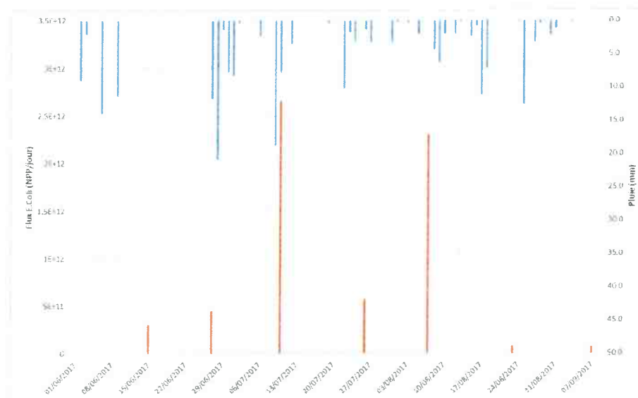
Figure 17 : Flux en E. coli du ru de Chantereine pendant l'été 2017 et cumul journalier de précipitations (pluviomètre GY28, DEA93).
