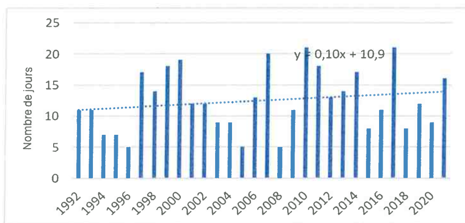
Figure 11 : Nombre de jours avec plus de 5 mm de pluie (juin-septembre, 1992-2021).
