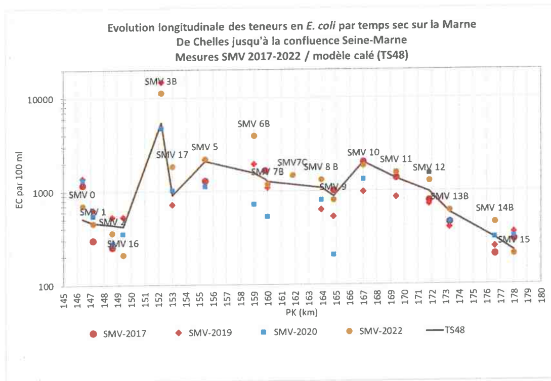
Figure 31 : Comparaison des résultats du modèle E. coli calé en temps sec aux données SMV
