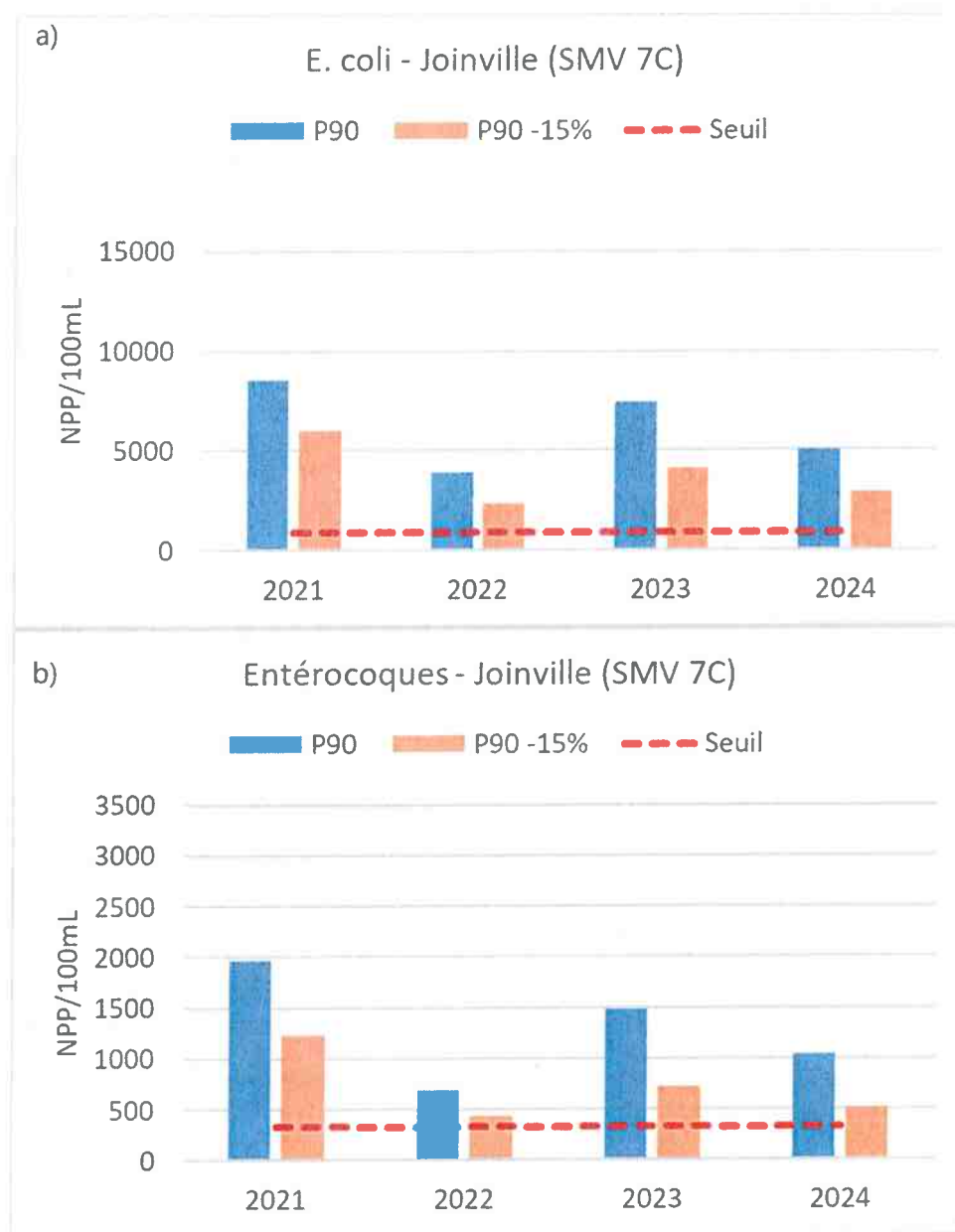
Figure 25 : Percentiles 90 des mesures en E. coli (a) et entérocoques (b) pour le site de Joinville-le-Pont de 2021 à 2024.
