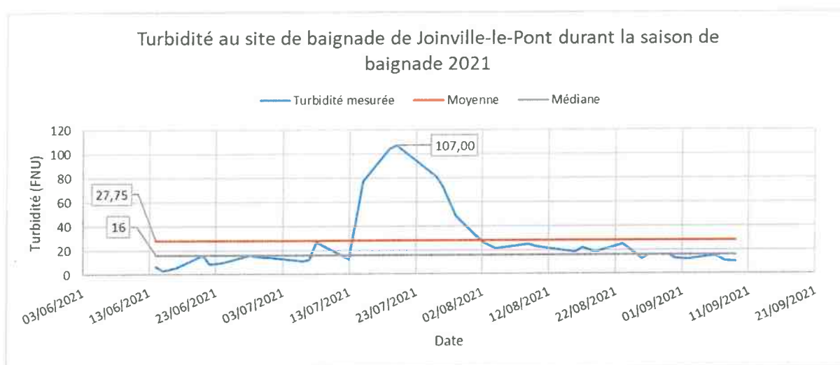
Figure 26 : Turbidité pendant la saison de baignade 2021 au site de Joinville-le-Pont.
