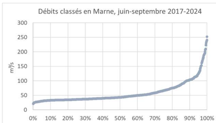
Figure 6 : Débits classés de la Marne sur la période estivale des années 2017 à 2024.
