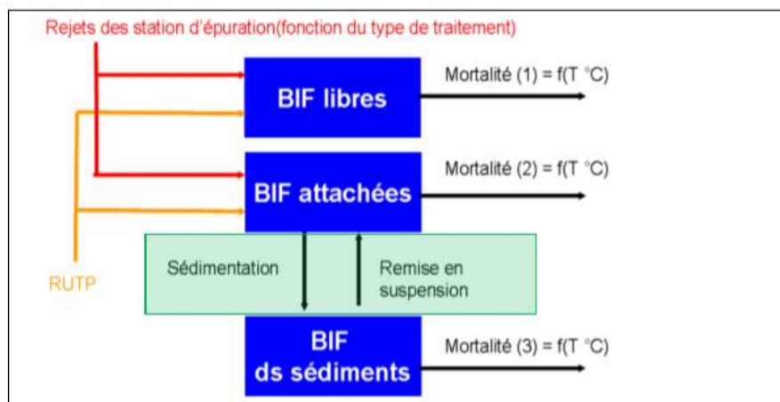
Figure 26 : Schéma des processus modélisés par WAQTEL.
