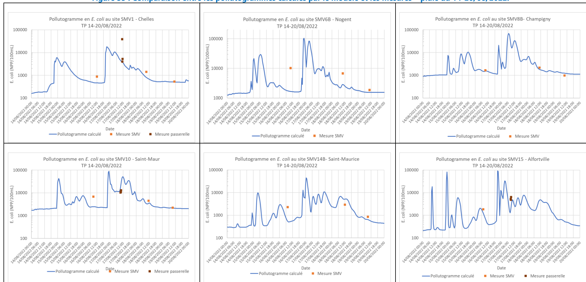
Figure 33 : Comparaison entre les pollutogrammes calculés par le modèle et les mesures – pluie du 14-20/08/2022.
