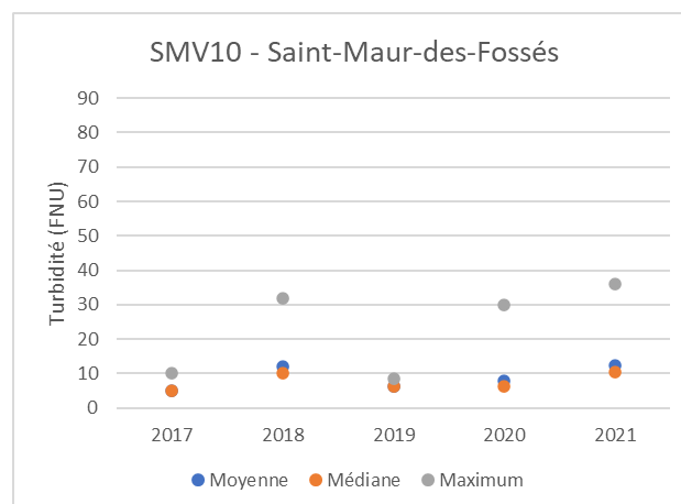
Figure 26 : Évolution de la turbidité pendant les saisons de baignade 2017 à 2021 au site de Saint-Maur-des-Fossés.
