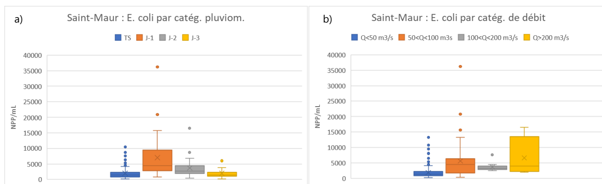
Figure 23 : Site de Saint-Maur-des-Fossés, boîtes à moustache des mesures en E. coli par contexte pluviométrique (a) et débitmétrique (b).
