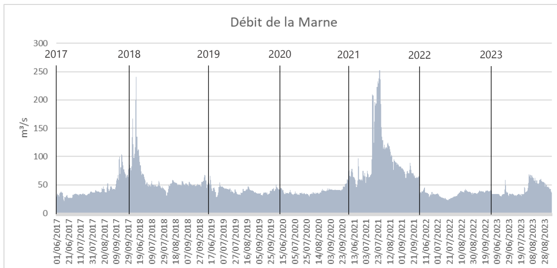
Figure 6 : Série des débits moyens journaliers mesurés en Marne sur la période estivale de 2017 à 2023.
