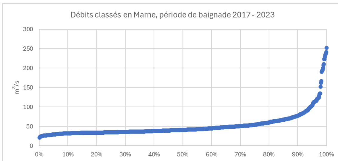
Figure 7 : Débits classés de la Marne sur la période estivale des années 2017 à 2023.
