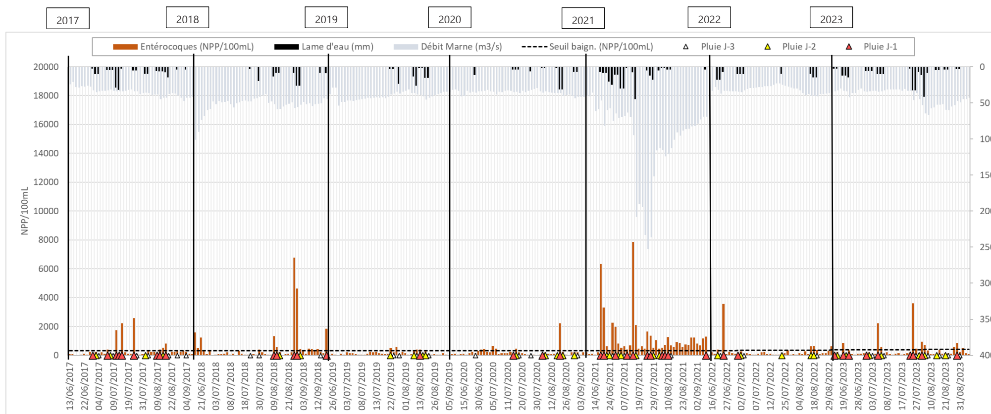
Figure 22 : Mesures en entérocoques au site de Saint-Maur-des-Fossés (SMV10) entre 2017 et 2023 ; axe secondaire : contexte pluviométrique et débitmétrique.
