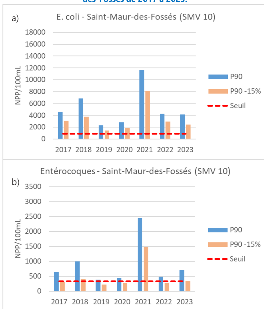
Figure 25 : Percentiles 90 des mesures en E. coli (a) et entérocoques (b) pour le site de Saint-Maur-des-Fossés de 2017 à 2023.
