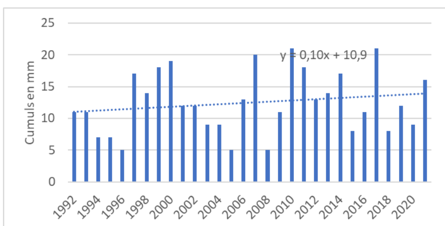
Figure 10 : Nombre de jours avec plus de 5 mm de pluie (juin-septembre, 1992-2021).
