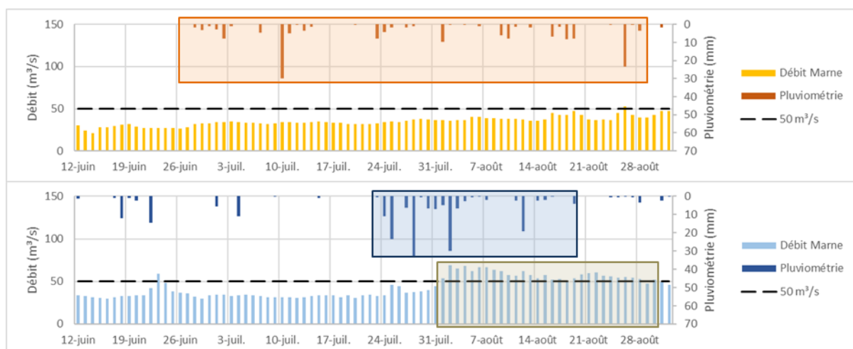
Figure 11 : Comparaison de la pluviométrie et des débits en 2017 et 2023.
