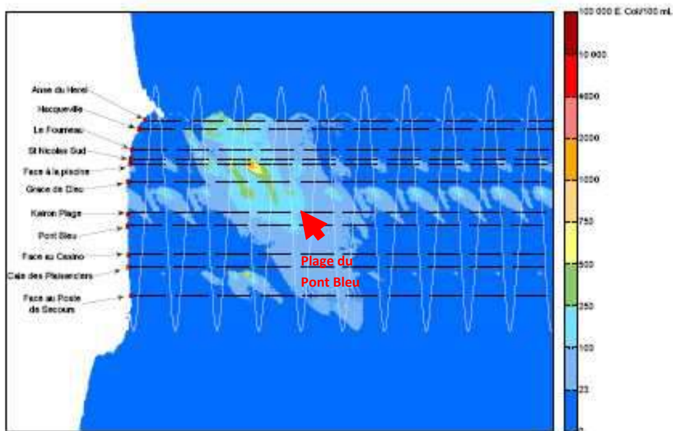
Figure 72 : Modélisation de la pollution microbiologique des fleuves côtiers et des émissaires pluviaux de la Baie GRANVILLE – JULLOUVILLE montrant l’impact de la Saigue plus spécifiquement– Projet Life Environnement Mareclean VERI 2009
