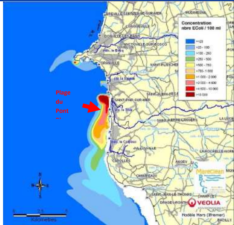
Figure 73 : Modélisation de l'impact du dysfonctionnement d'un ouvrage d'assainissement implanté sur le bassin versant du Thar – Projet Life Environnement Mareclean VERI 2009
