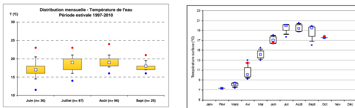
Figure 13a et b: Distribution mensuelle de la température de l'eau sur la période estivale 1997-2010 (DT50-ARS BN) - Distribution mensuelle de la température de surface à Granville sur la période 2003-2006 (IFREMER-LERN)
